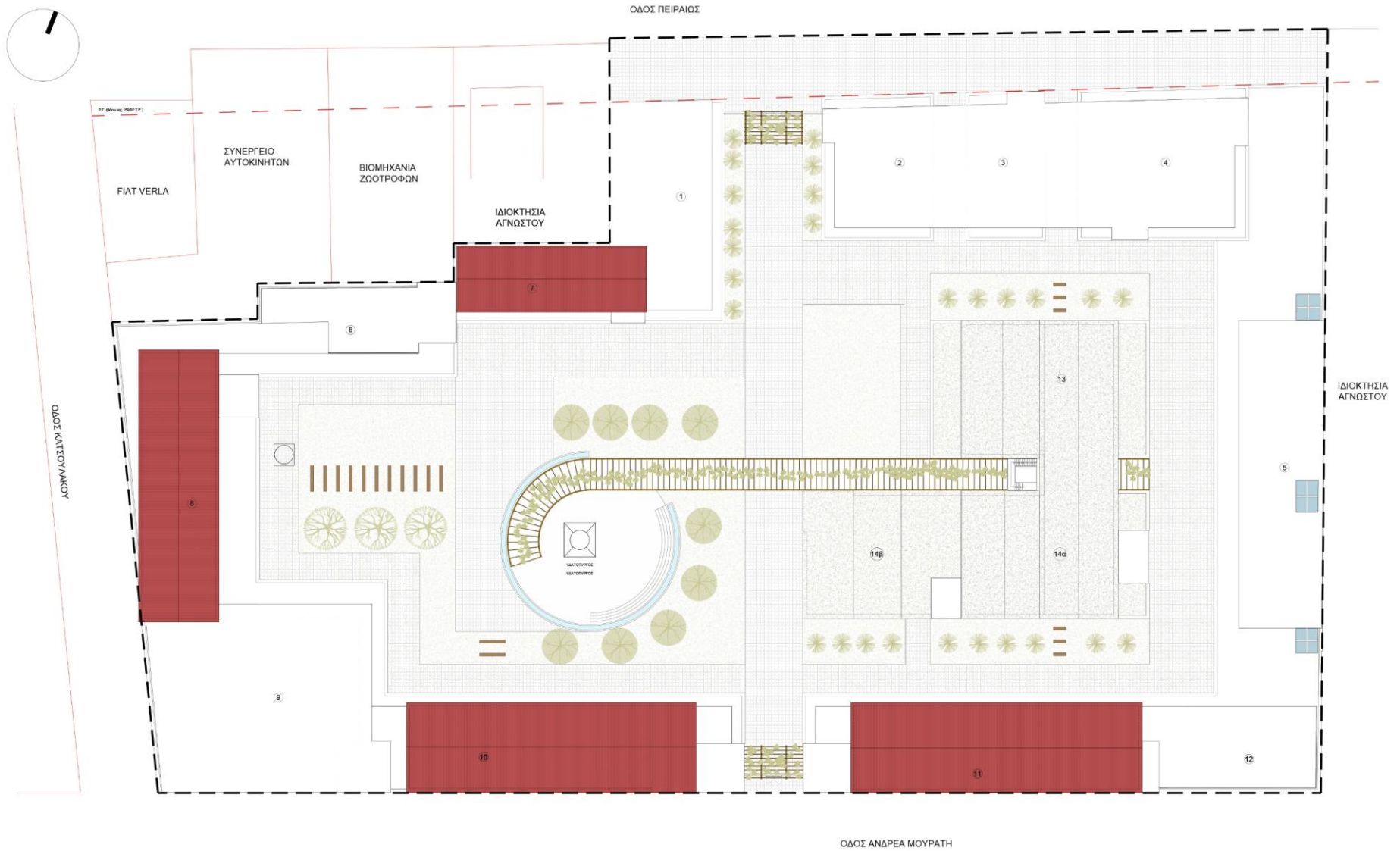
Κάτοψη Στεγών
